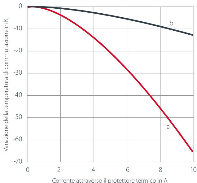
Fig. 2: riscaldamento proprio della corrente: comportamento tipico di un protettore termico sensibile ad alta intensità di corrente con disco bimetallico (a) sotto tensione (a) rispetto a protettori termici con disco bimetallico non sotto tensione (b)
