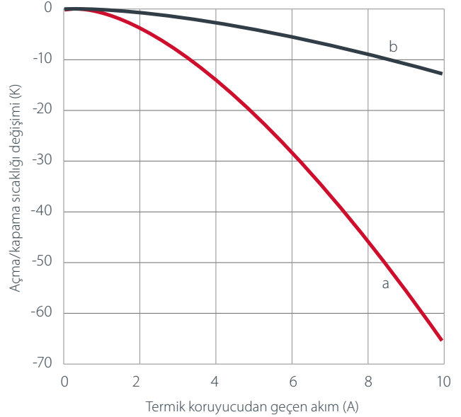
Şek.2: Akım ile ısınan: akım taşıyan bimetal diske sahip yüksek akıma duyarlı termal koruyucu (a) ile akım taşıyan bimetal diske sahip olmayan termal koruyucuların tipik davranışlarının karşılaştırması (b)
