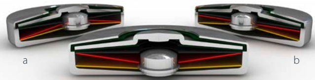
Şek. 2: Ek esnek diskli (sarı) termik koruyucunun işlevi ve açma/kapama davranışı, bu sayede bimetal disk (kırmızı) sürekli çalışabilmektedir.
