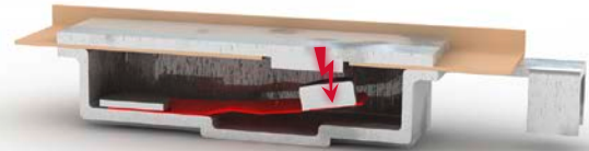
Şek.3: Ekstra esnek disk olmayan termik koruyucu. Bundan dolayı oluşan ark hasarı riski.
